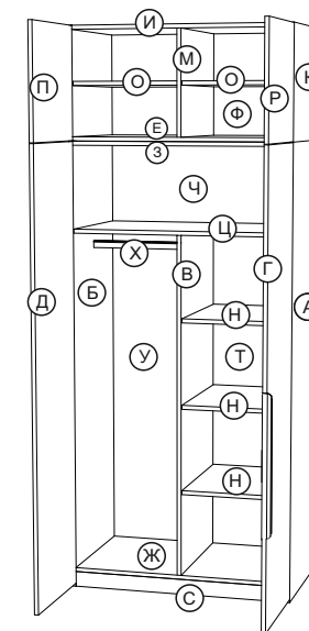
Модуль М25 Д*В*Г 1000*2500*600
